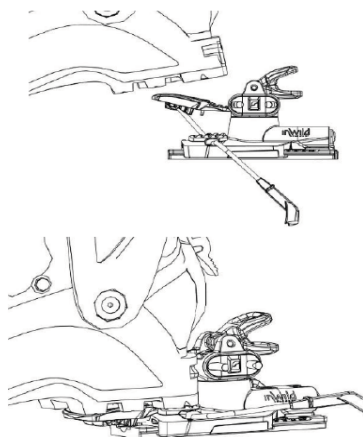
Verrouillage du stop-ski pour la montée
