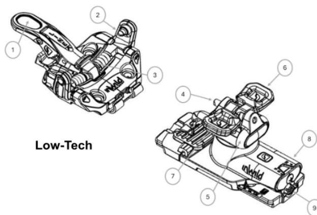
Heel support
