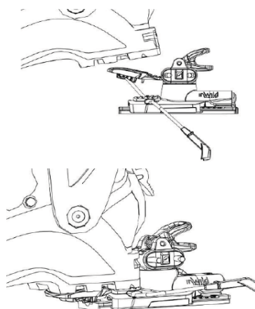
Verriegelung der Skistoppers beim Bergsteigen (Lauf-modus)
