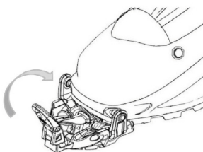
Laufstelle (Verriegelungshebel angehoben)
